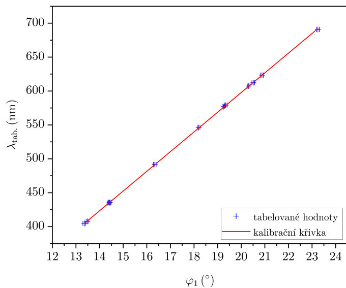
Graf 1: Kalibrační křivka spektrometru
