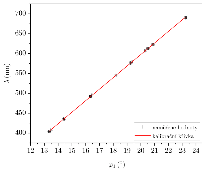
Graf 2: Proložení naměřených hodnot kalibrační křivkou
